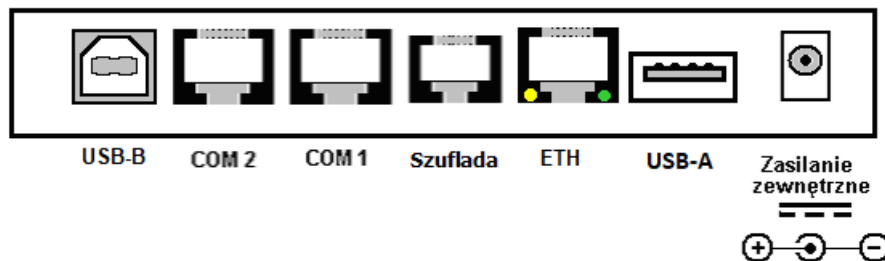
Rys. 6.1a. Widok panelu gniazd zewnętrznych
