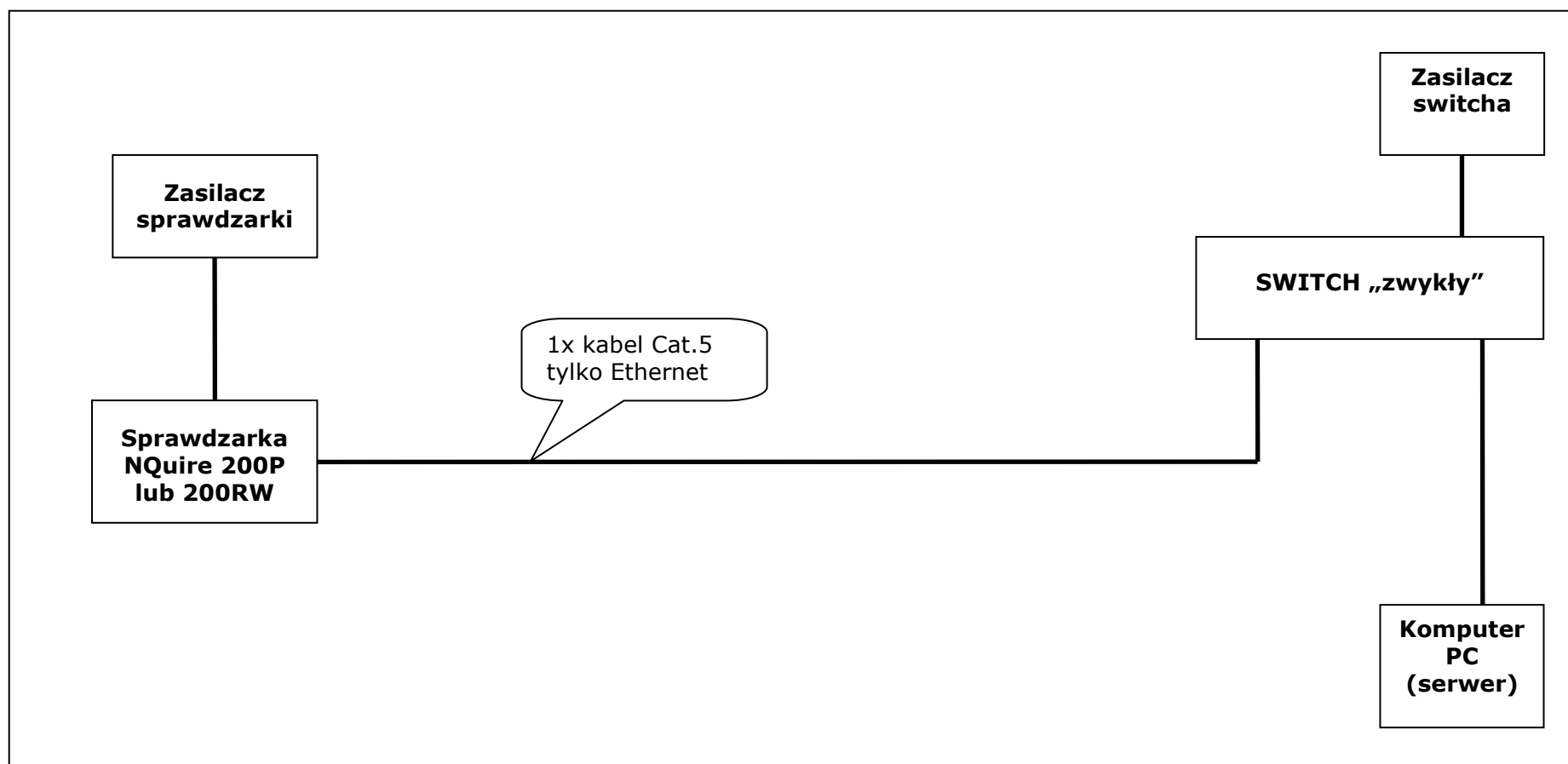
Przykład 1. Lokalne zasilanie sprawdzarki
